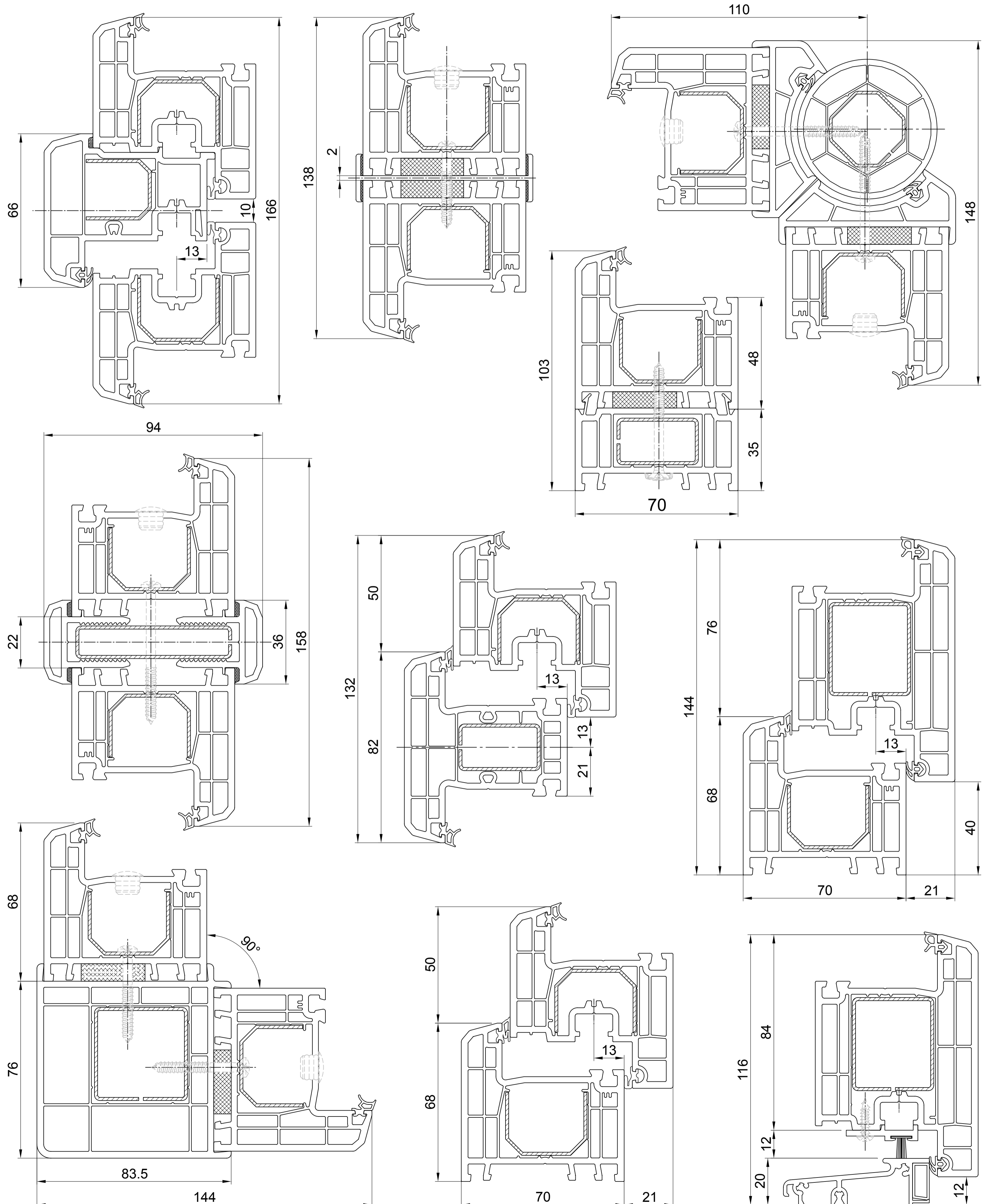
59-03 соединитель импоста (пластик)
