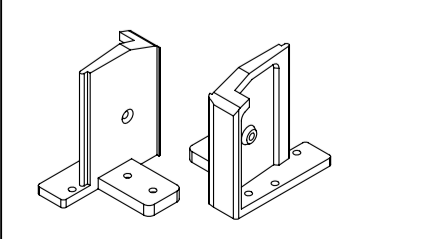
59-05 соединитель порога ширина 70мм
